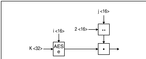
Figure 7-289. Compute XTS Parameter Using AES 256
