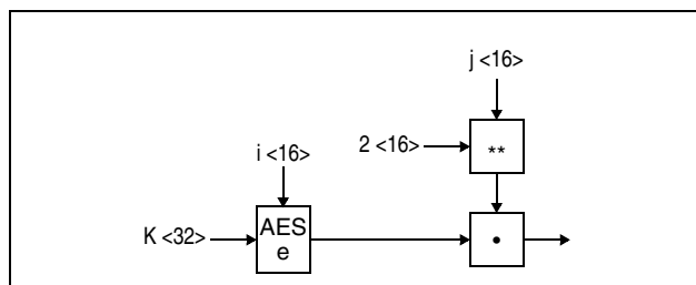
Figure 7-288. Compute XTS Parameter Using AES 256
