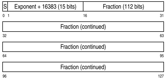
Figure 19-3. BFP Extended Format (16 bytes)
