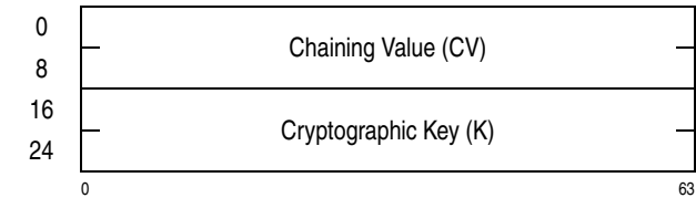
Figure 7-160. Parameter Block for KMO-AES-128
