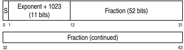
Figure 19-2. BFP Long Format (8 bytes)
