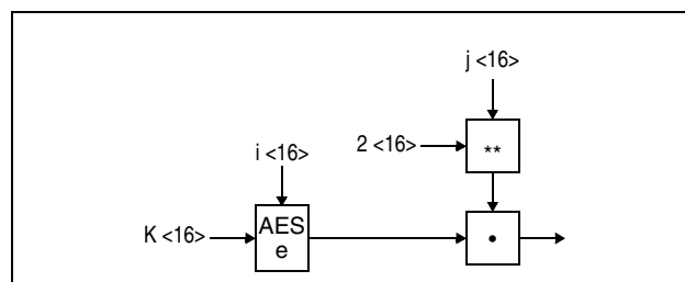
Figure 7-285. Compute XTS Parameter Using AES 128
