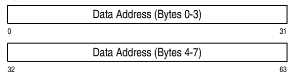
Format-2 IDAW
